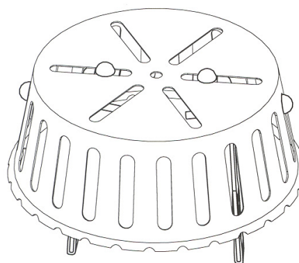
Crépine moulée
