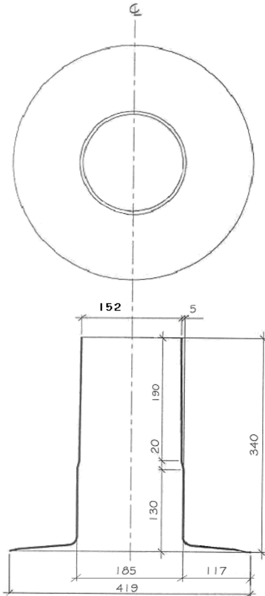
Manchon d'évent 6'' (152.4 mm)
