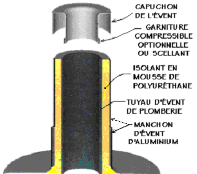
Section d'évent
