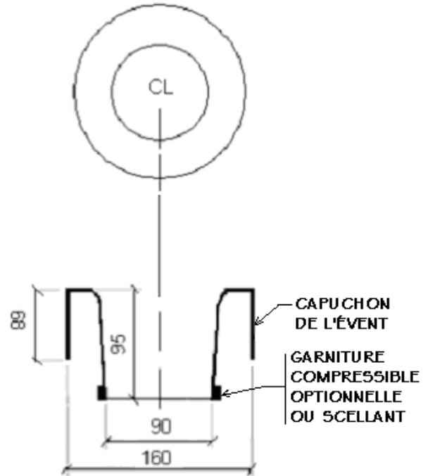
Capuchon d'évent
